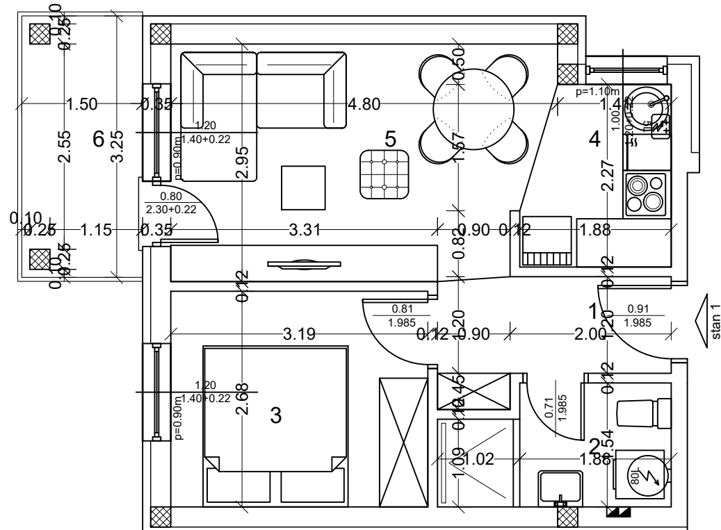
OSNOVA STANA BR. 1, P=37,04 m 2
