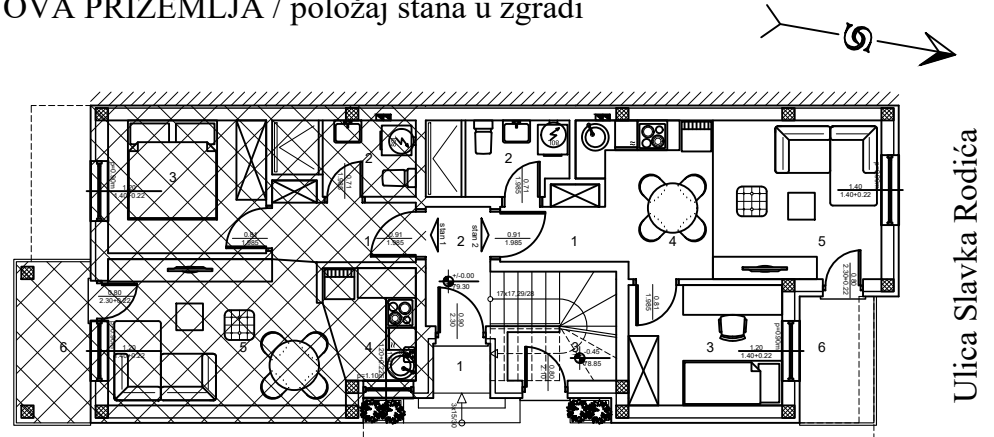
OSNOVA PRIZEMLJA / položaj stana u zgradi
