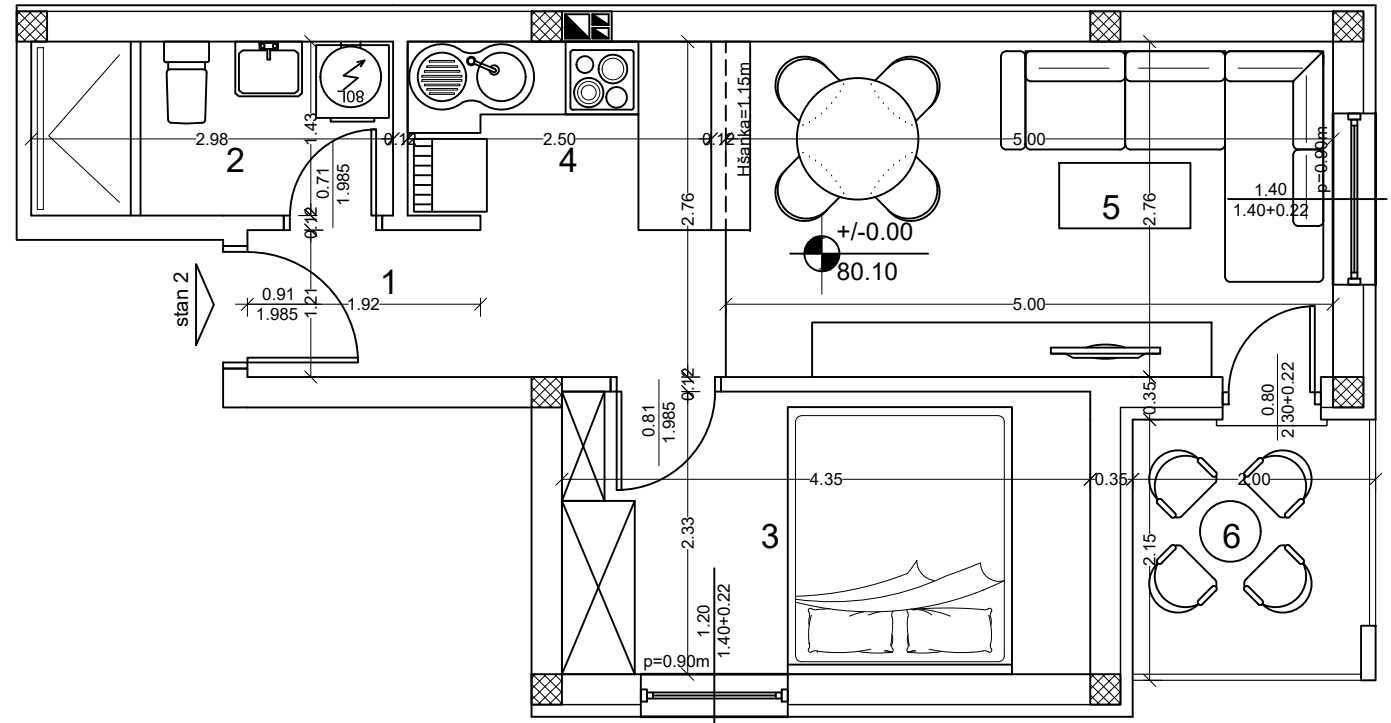
OSNOVA STANA BR. 2, P=39,62 m 2
