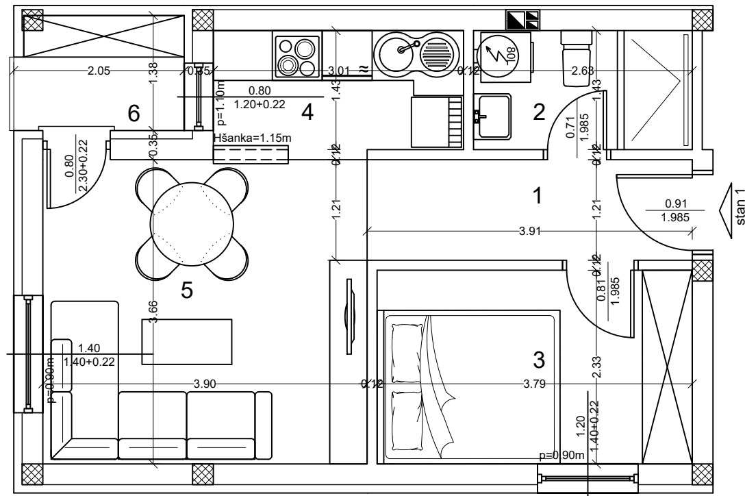
OSNOVA STANA BR. 1, P=37,71 m 2
