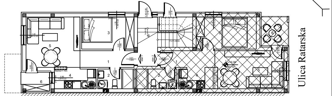
OSNOVA PRIZEMLJA / položaj stana u zgradi
